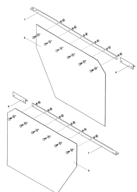
ETB-007852, Osłona przeciwbłotna
