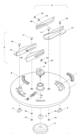
ETB-007837, Tarcze do rozsiewu granicznego TS 10-14 ZA-M Special
