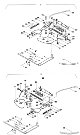
ETB-007844, Płyta denną z zasuwą ZA-M Special
