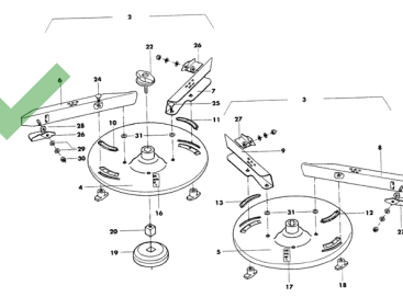
ETB-007835, Tarcze rozsiewające OS 20-28 ZA-M Special
