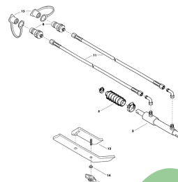
ETB-007849, Siłownik hydr. pojedynczej zasuwy dwustronnego działania ZA-M Special
