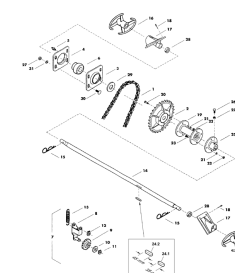
ETB-007843, Wałek mieszadła i jarzmo napinające do łańcucha
