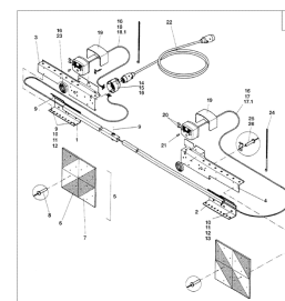
ETB-007854, Instalacja
