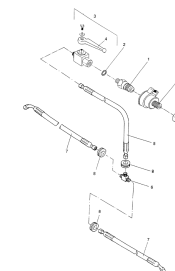
ETB-007847, Siłownik hydr. podwójnej zasuwy ZA-M Special
