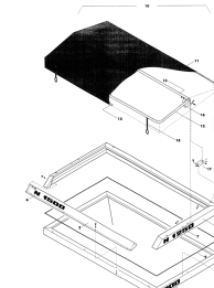
ETB-007851, Nadstawka nad zbiornik N i składana plandeka ZA-M Special
