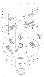
ETB-007836, Tarcze do rozsiewu granicznego TS 5-9 ZA-M Special
