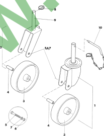
ETB-007853, Urządzenie
