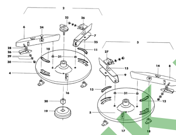
ETB-007834, Tarcze rozsiewające OS 10-18 ZA-M Special
