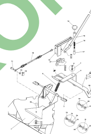
ETB-007838, Ekran rozsiewu granicznego z obu stron ze zdalnym sterowaniem ZA-M Special
