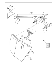
ETB-007839, Ekran rozsiewu granicznego ZA-M Special
