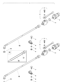
ETB-007848, Siłownik hydr. pojedynczej zasuwy jednostronnego działania ZA-M Special
