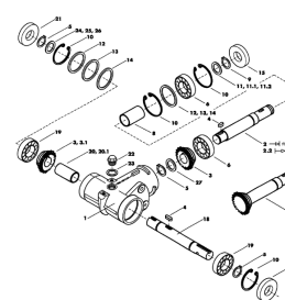
ETB-007842, Przekładnia wejściowa i specjalna przekładnia
